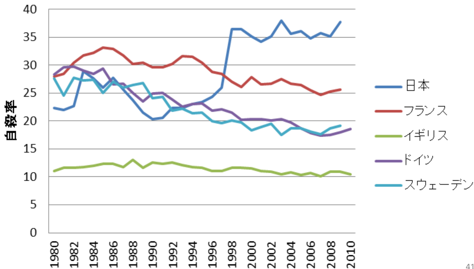
自殺率の年次推移 (男性)
